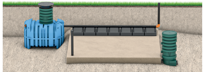
Markbaserad markbädd vid lerig mark
