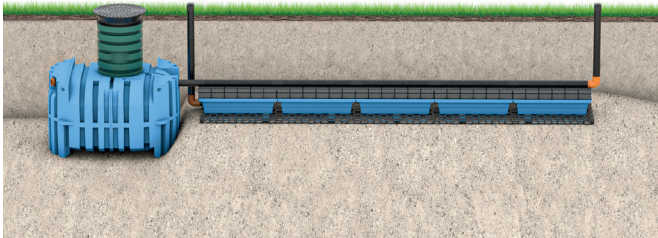
Markbaserad infiltration vid jordig/sandig mark
