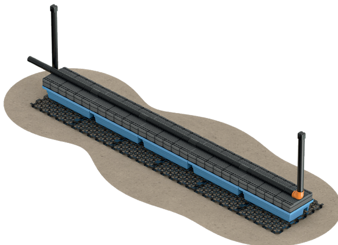
Exempel på infiltration med FANN INDRÄN® Plus Biomoduler
