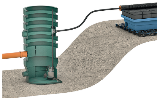
Illustration av pumpning med pumpbrunn
