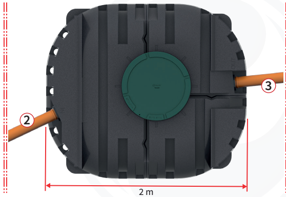
PLANSEKTION
